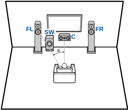
a: 22°至 30°
